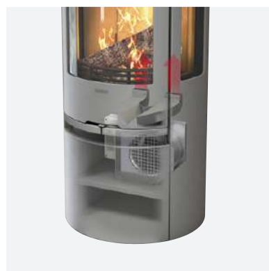
Ventilateur Assure une répartition rapide de la chaleur et une température uniforme. Régulation thermostatique assurant un démarrage automatique au moment de l'allumage et l'arrêt quand le feu s'éteint. Ce ventilateur est facile à monter même après coup.
